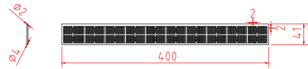
integrierter Insektenschutz für Lamelle 45 aus Kunststoff (PB1)
