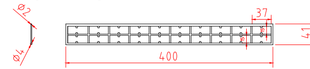
integrierter Vogelschutz für Lamelle 45 aus Kunststoff (PB1)
