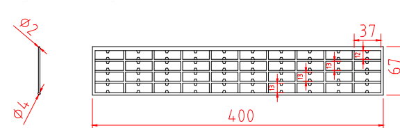
integrierter Vogelschutz für Lamelle 75 aus Kunststoff (PB1)
