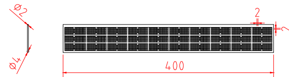
integrierter Insektenschutz für Lamelle 60 aus Kunststoff (PB1)
