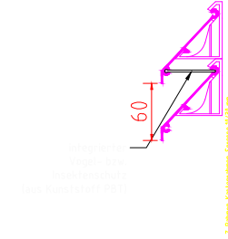
BEISPIEL Lamelle 60 mit integriertem Vogel/Insekten- schutzgitter
