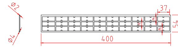
integrierter Vogelschutz für Lamelle 60 aus Kunststoff (PB1)
